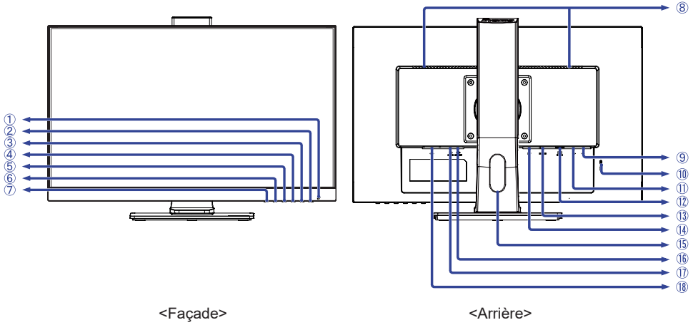
<Façade>
